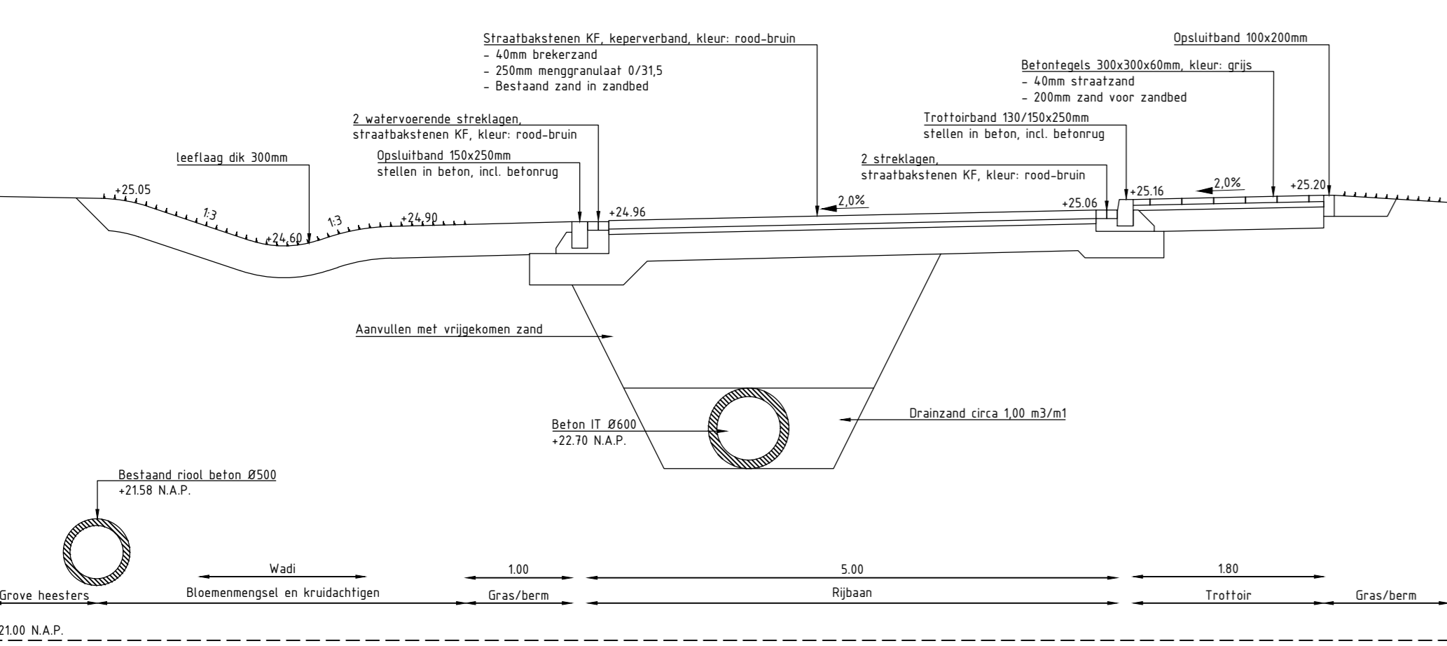
Dwarsprofiel A-A Schaal 1: 50
