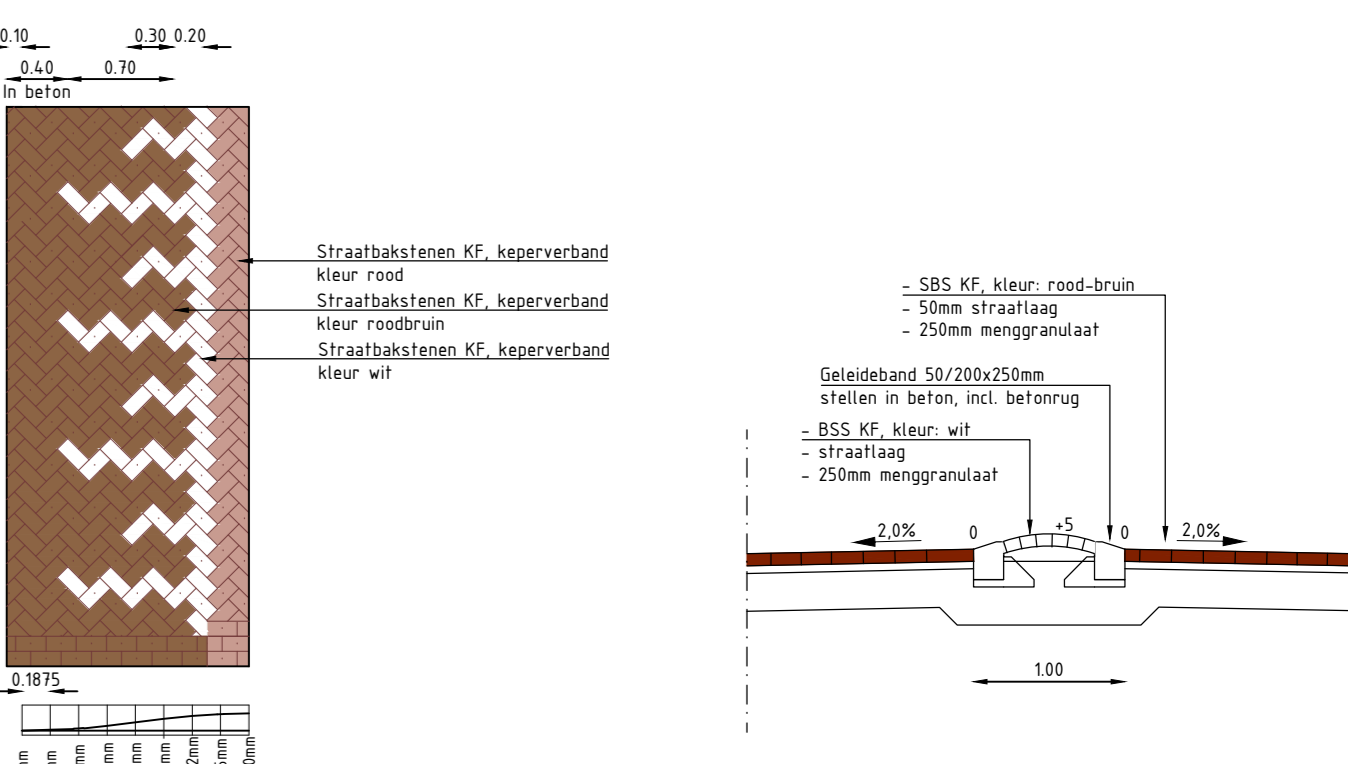
Principedetail talud verkeersplateau Detail 1: 'bol' straten middengeleider
