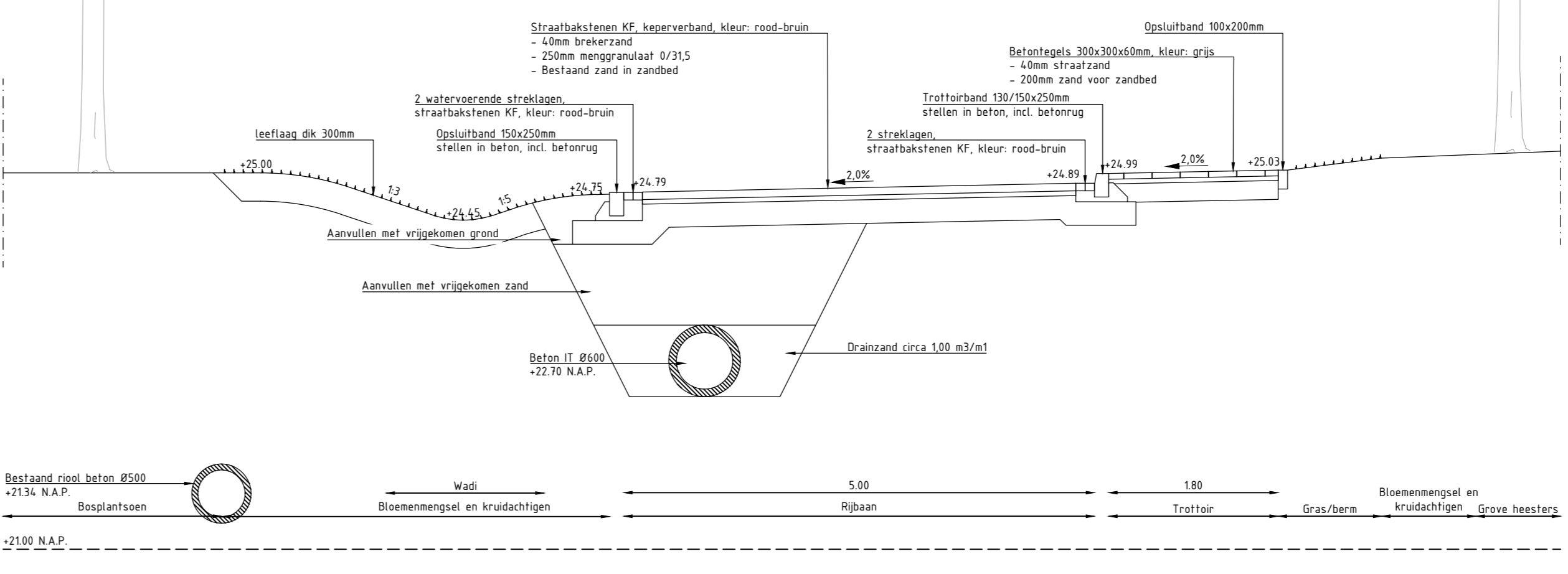
Dwarsprofiel C-C Schaal 1: 50
